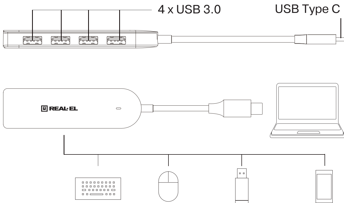
Схема подключения
